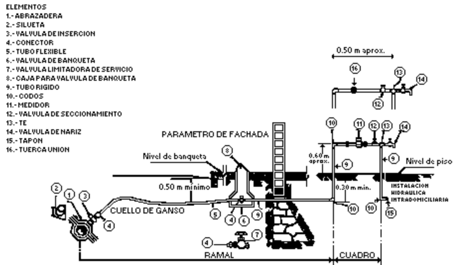
FIGURA No. 1 TOMA DOMICILIARIA CON VALVULA DE BANQUETA
