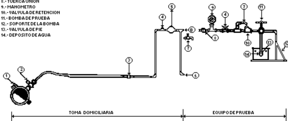
FIGURA No. 6 ESQUEMA DE PRUEBA DE LA TOMA DOMICILIARIA, CON EQUIPO DE PRUEBA
