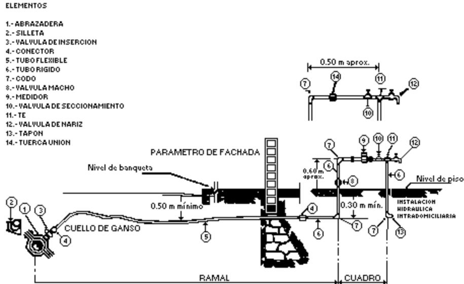
FIGURA No. 2 TOMA DOMICILIARIA SIN VALVULA DE BANQUETA
