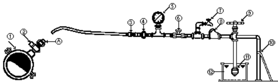
FIGURA No. 5 ESQUEMA DE PRUEBA DE ABRAZADERA/SILETA Y VALVULA DE INSERCIION
